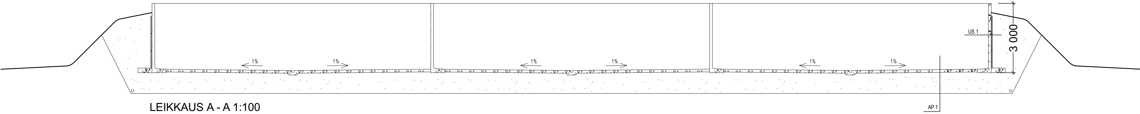
LEIKKAUS A - A 1:100
