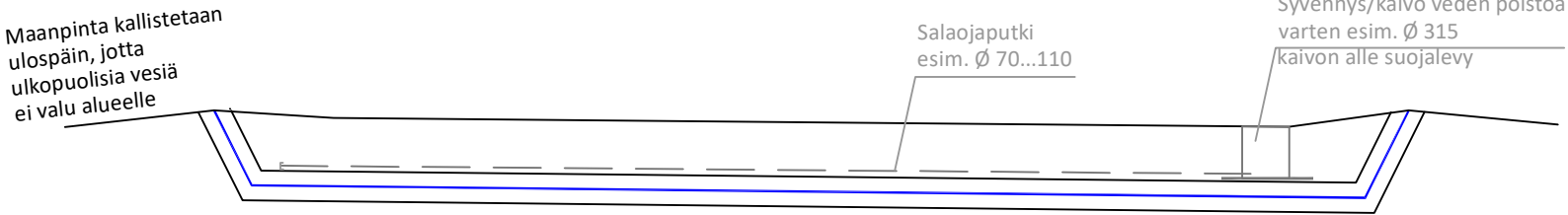
LEIKKAUS A-A
