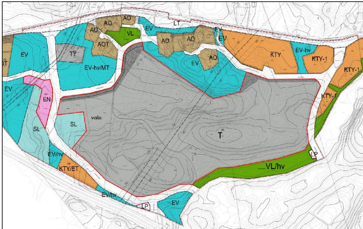
Etelä-Nummelan työpaikka-alue I asemakaava
