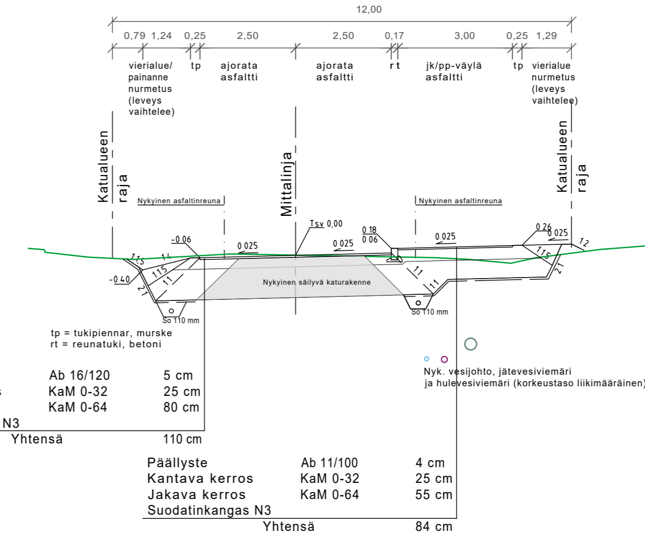
Tyypipokkileikkaus 1:100 Kotikyläntie
