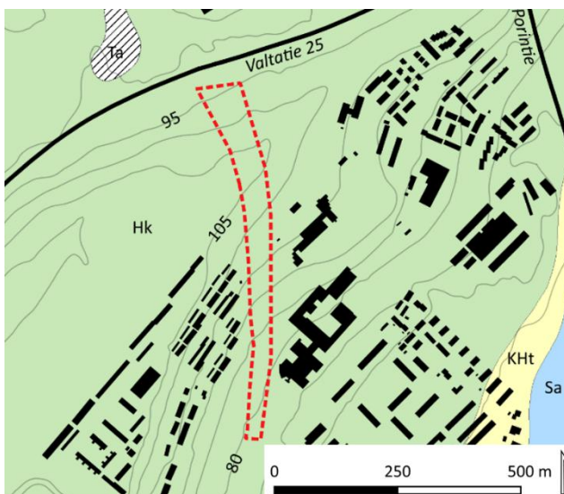
Kuva 5. Suunnittelualueen maaperä ja topografia. Hk=Hiekka, Kht=Karkea hieta, Sa=Savi, Ta=Täytemaa. Suunnittelualueen raja- aus on punaisella katkoviivalla ja rakennukset mustalla. (Maaperä © GTK, Maastotieto- kanta (muokattu) © Maanmittauslaitos 05/2025).
