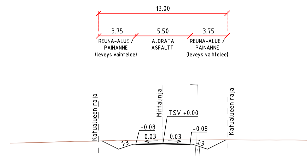
TYYPPIPOIKKILEIKKAUS H-H 1:200
