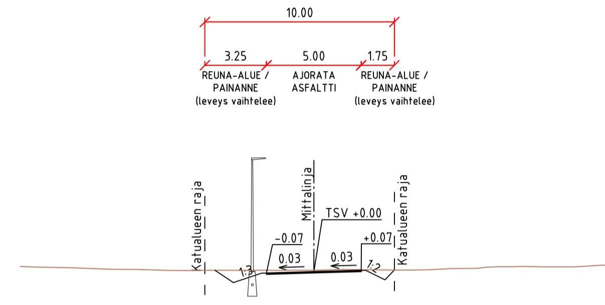
TYYPPIPOIKKILEIKKAUS G-G 1:200
