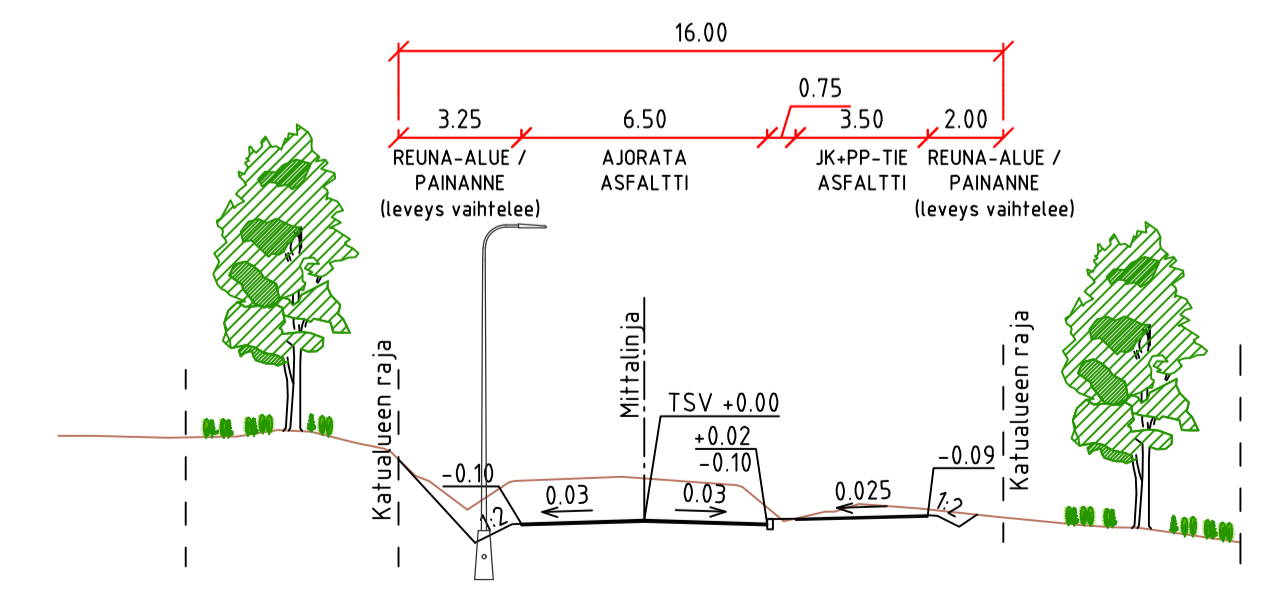
TYYPPIPOIKKILEIKKAUS C-C 1:200
