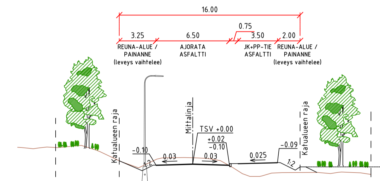
TYYPPIPOIKKILEIKKAUS B-B 1:200
