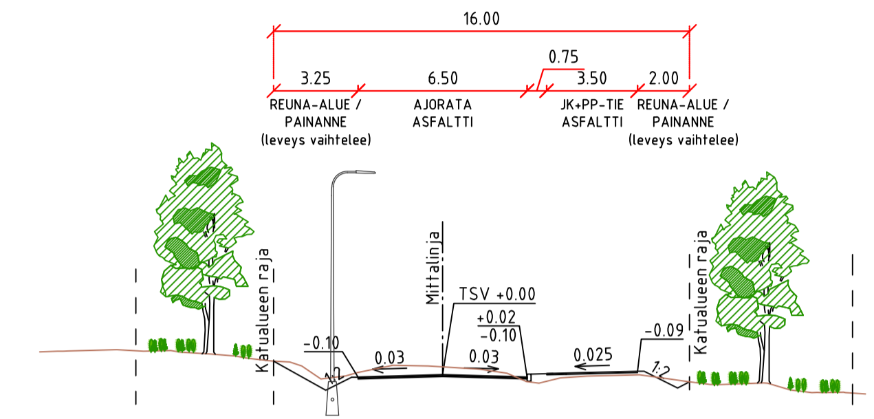
TYYPPIPOIKKILEIKKAUS A-A 1:200
