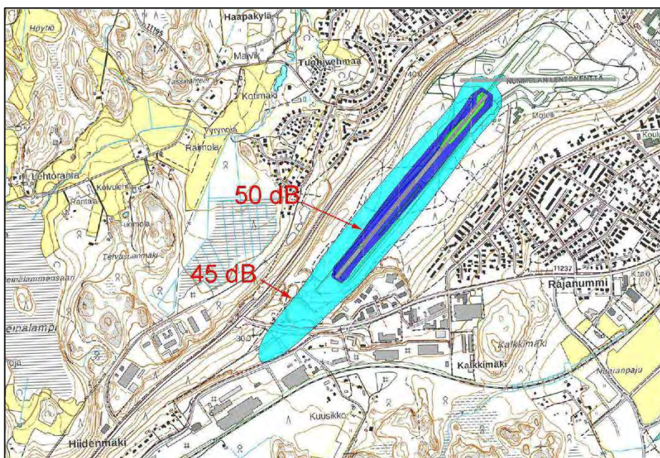
Kuva 9. Melun keskiäänitaso, yöaika (22–07). Nummelan lentokenttä EFNU, Äänitasomallinnus päivitys 13.11.2022, Windcraft Oy.
