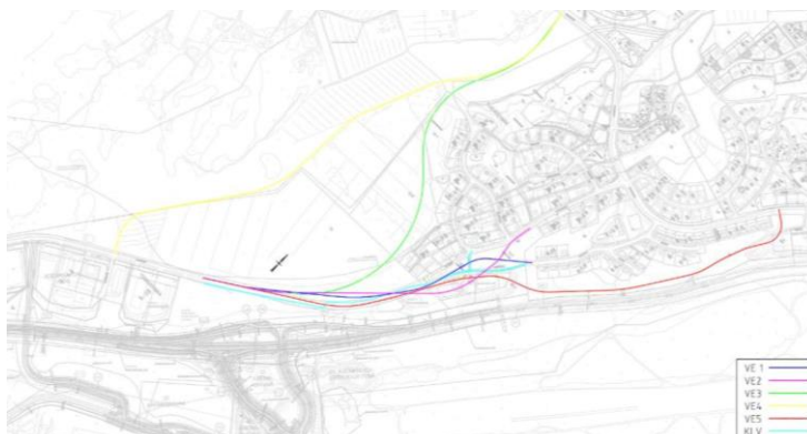
Kuva 48. Uuden kokoojakatuyhteyden linjausvaihtoehdot. (FCG, 2023)
