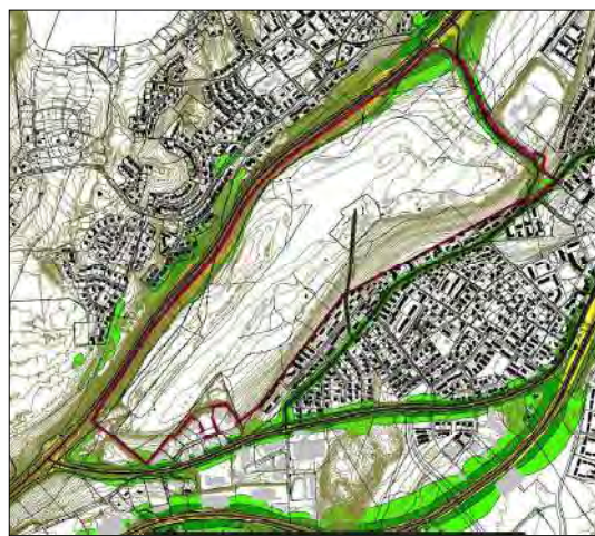
Tieliikennemelut, yöaika, 2023
