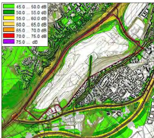
Tieliikennemelut, päiväaika, 2023
