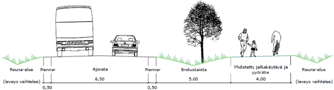
Kuva 13 Hankasalontien tyypipiikkileikkaus.
