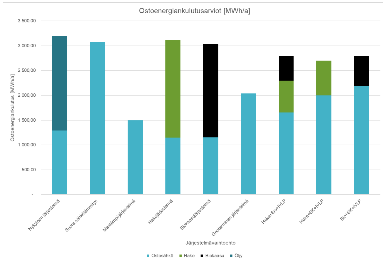
Kuva 15. Järjestelmävaihtoehtojen ostoenergiankulutusarvio.
