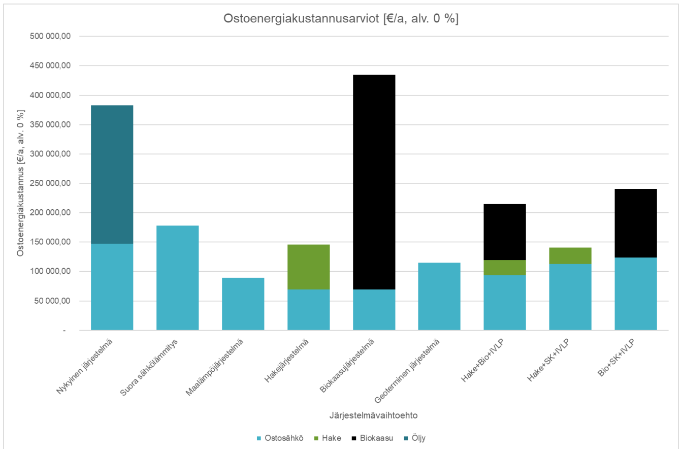
Kuva 16. Järjestelmävaihtoehtojen ostoenergiakustannusarvot.
