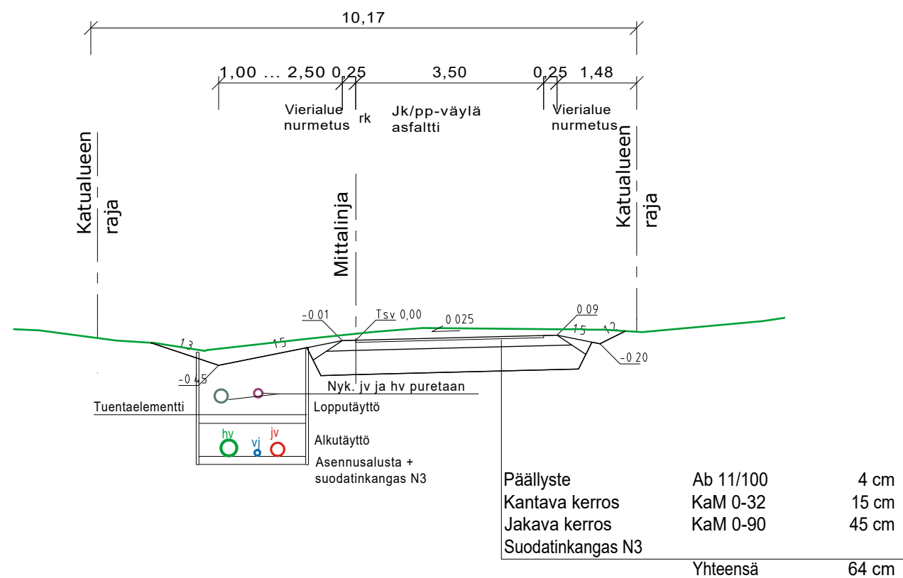
TYYPPIPOIKKILEIKKAUS 1:100 Rinnepolku
