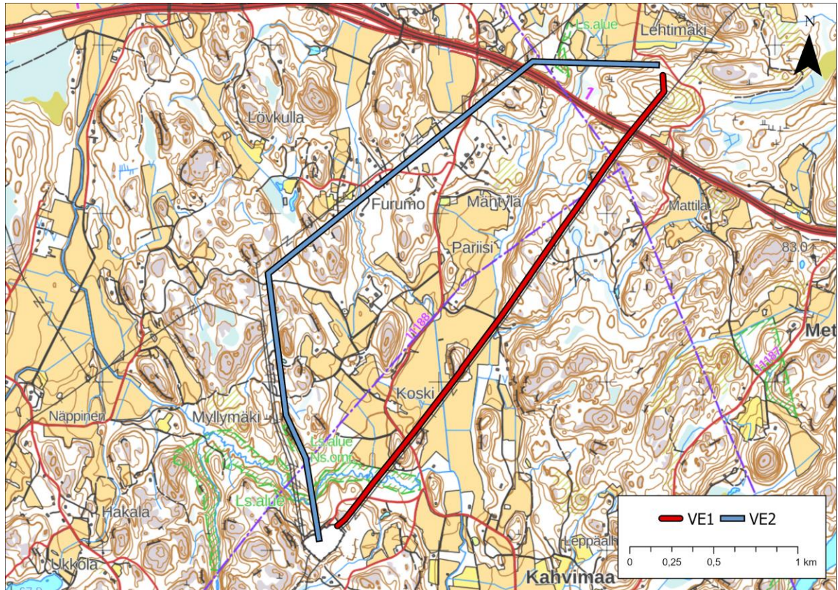
Kuva 2-3 Esisuunnittelussa tarkastellut vaihtoehtoiset voimajohtoreitit: eteläinen reittivaihtoehto VE1, jossa 2x110 kV voimajohto toteutettaisiin olemassa olevan 400 kV:n voimajohdon rinnalle punaisen linjan mukaisesti sekä pohjoinen reittivaihtoehto VE2, jossa toinen 110 kV voimajohto kulkisi lännempänä, olemassa olevan 110 kV:n voimajohdon rinnalla (sininen) ja toinen 110 kV voimajohto kuten vaihtoehdossa VE1 olemassa olevan 400 kV:n voimajohdon rinnalla (punainen).
