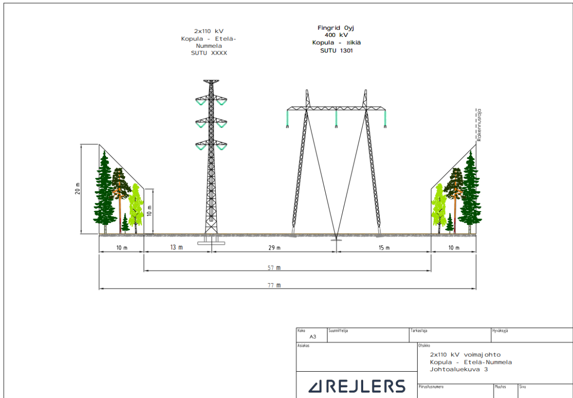
Kuva 2-4. 2x110 kV voimajohdon tilantarve yhdistetyssä maastokäytävässä Fingrid Oyj:n Kopula – Hikiä (SUTU 1301) 400 kV voimajohdon rinnalla. (Kuva: Rejlers)
