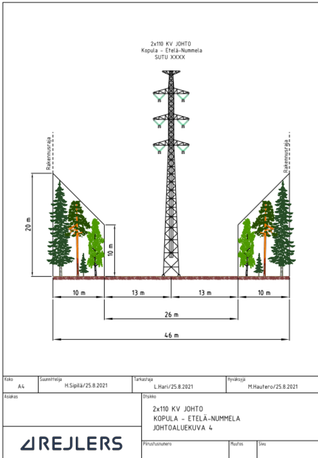
Kuva 2-5 2x110 kV voimajohdon tilantarve omassa maastokäytävässä (VE1b mukainen toteutus alueella, jossa johto ei sijoitu olemassa olevan Fingrid Oyj:n Kopula – Hikiä (SUTU 1301) 400 kV voimajohdon rinnalle. (Kuva: Rejlers)
